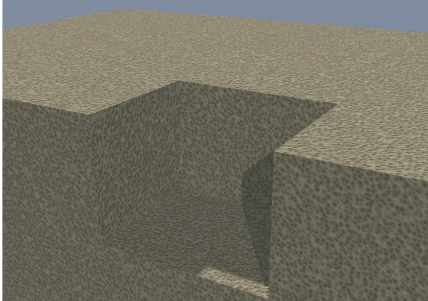
Schritt 1. Baugrube 200 × 160 cm, Tiefe 145 cm
