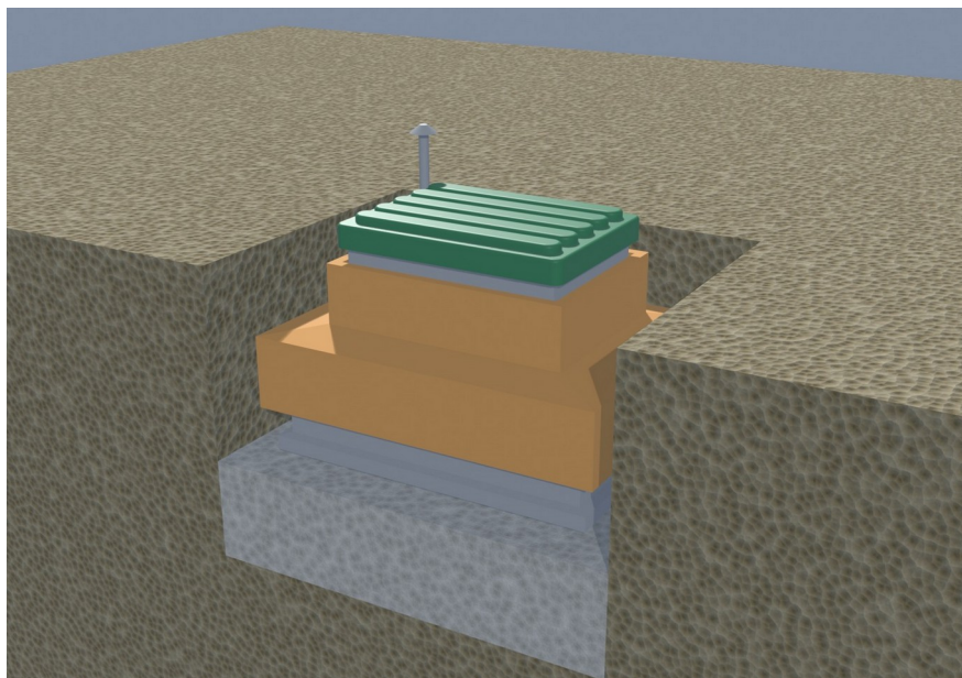
Schritt 6. Dämmung von Einstieg, Oberseite und Wänden auf 30 cm, XPS 5 cm
