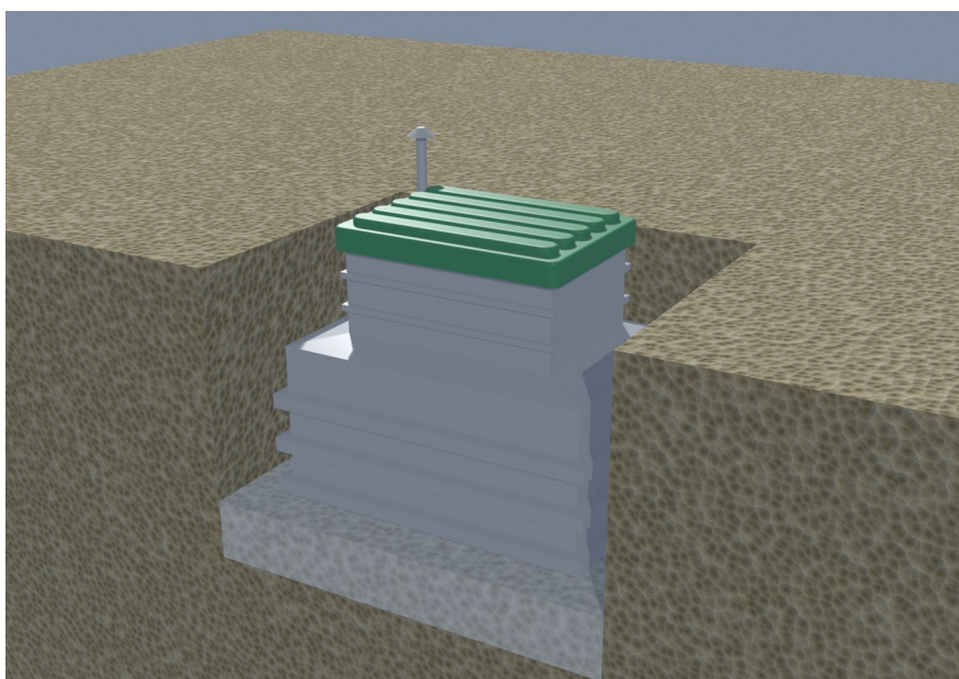
Schritt 5. Erste Trockenbetonlage, 20 cm
