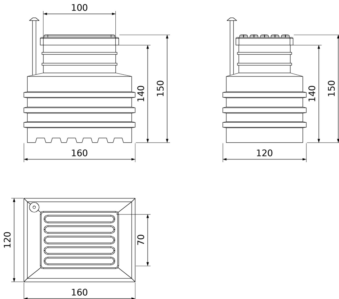
Gartenkeller 120 × 160 — drei Ansichten, Maße in Zentimetern
