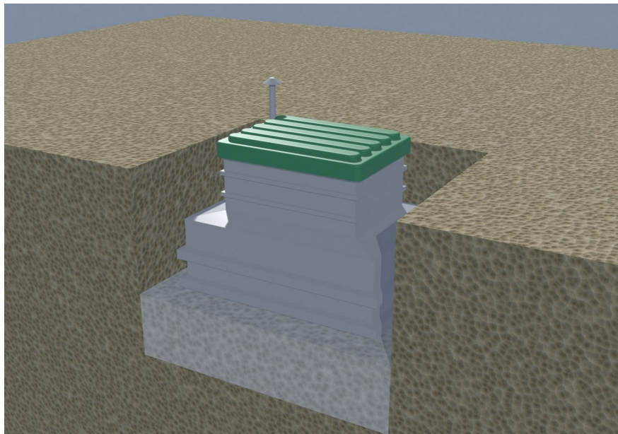
Schritt 5. Umfüllung mit Trockenbeton bis 40 cm Höhe
