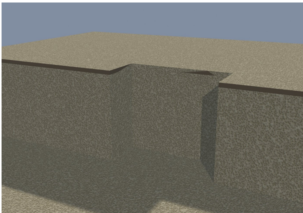
Schritt 1. Baugrube 240 × 240 cm, Tiefe 268 cm, und Aushub für den Schacht
