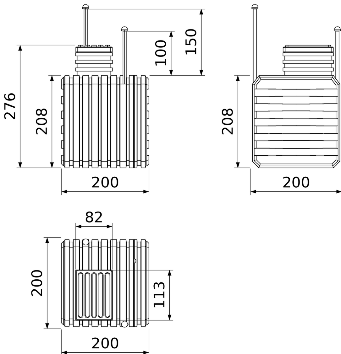
Gartenkeller 200 × 200 — drei Ansichten, Maße in Zentimetern
