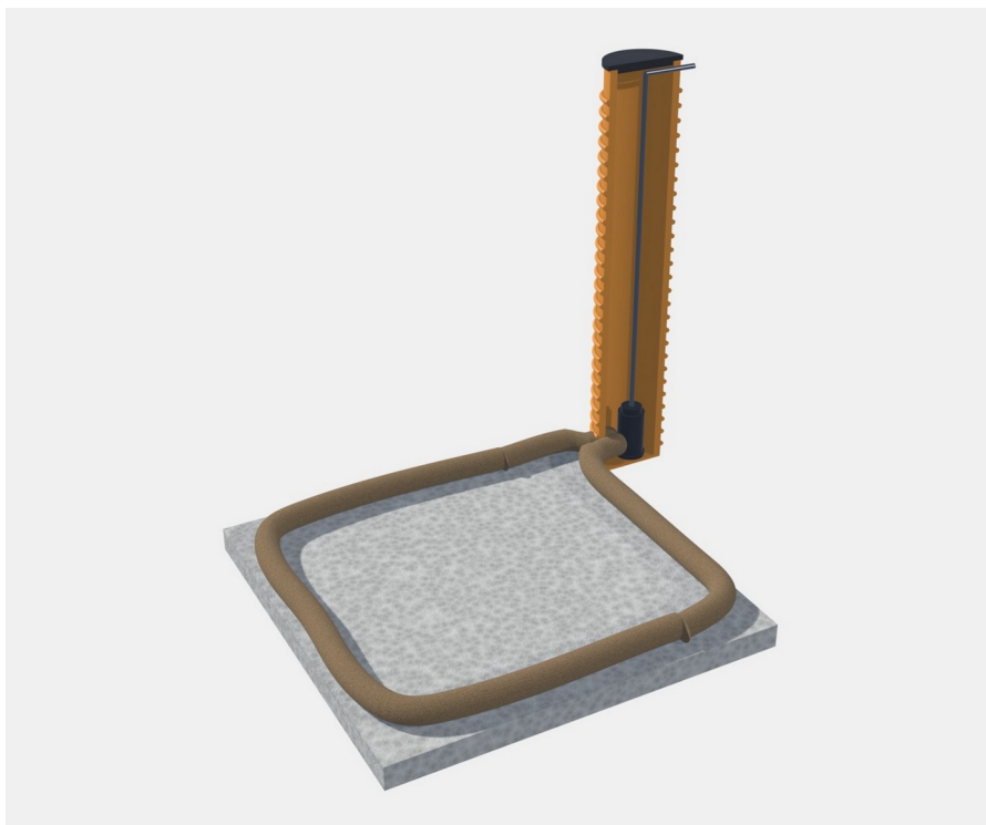
Schema des Drainagesystems: Bodenplatte, Ringröhr, Schacht im Schnitt, Pumpe und Druckleitung
