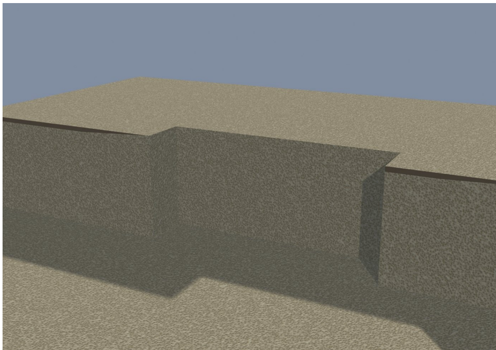
Schritt 1. Baugrube 520 × 240 cm, Tiefe 268 cm, und Aushub für den Schacht
