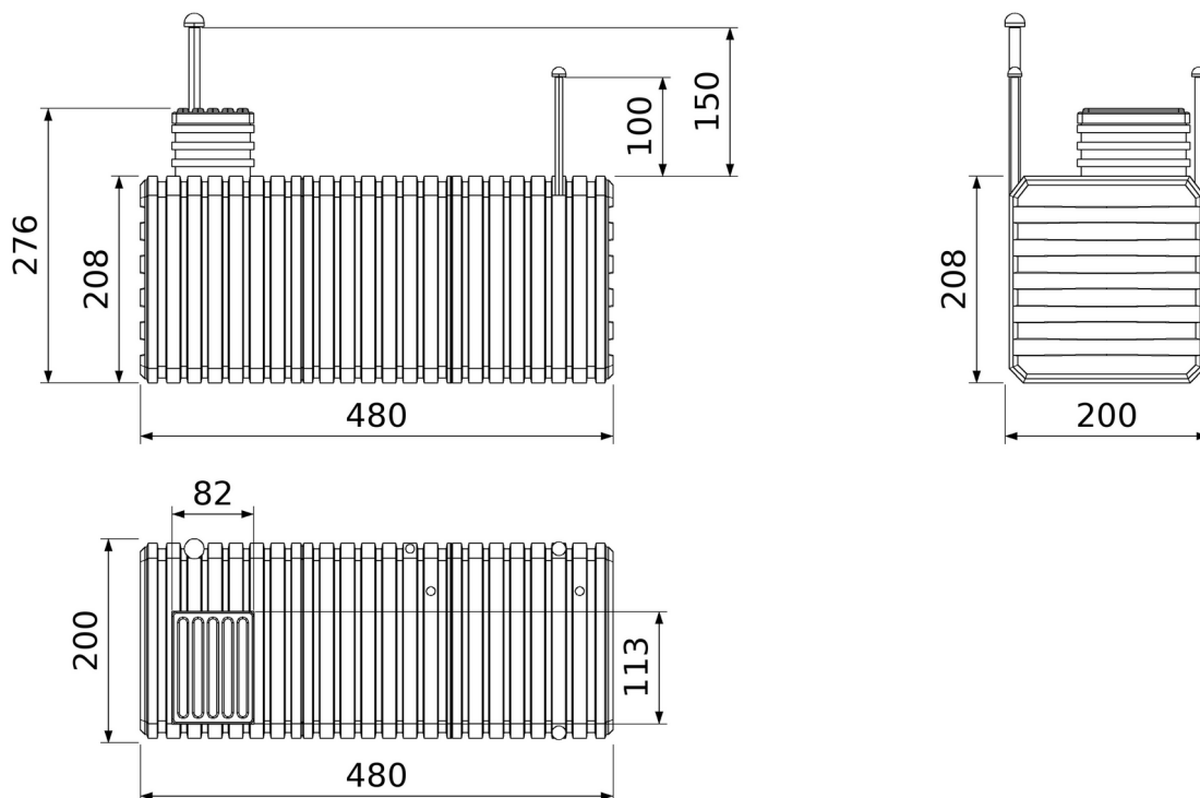
Gartenkeller 200 × 480 — drei Ansichten, Maße in Zentimetern
