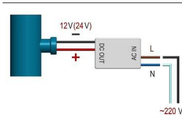
Anschlussschema der Beleuchtung: Kabelführung über Abzweig 100 × 50 × 100 mm, Netzteil 220 / 12 V
